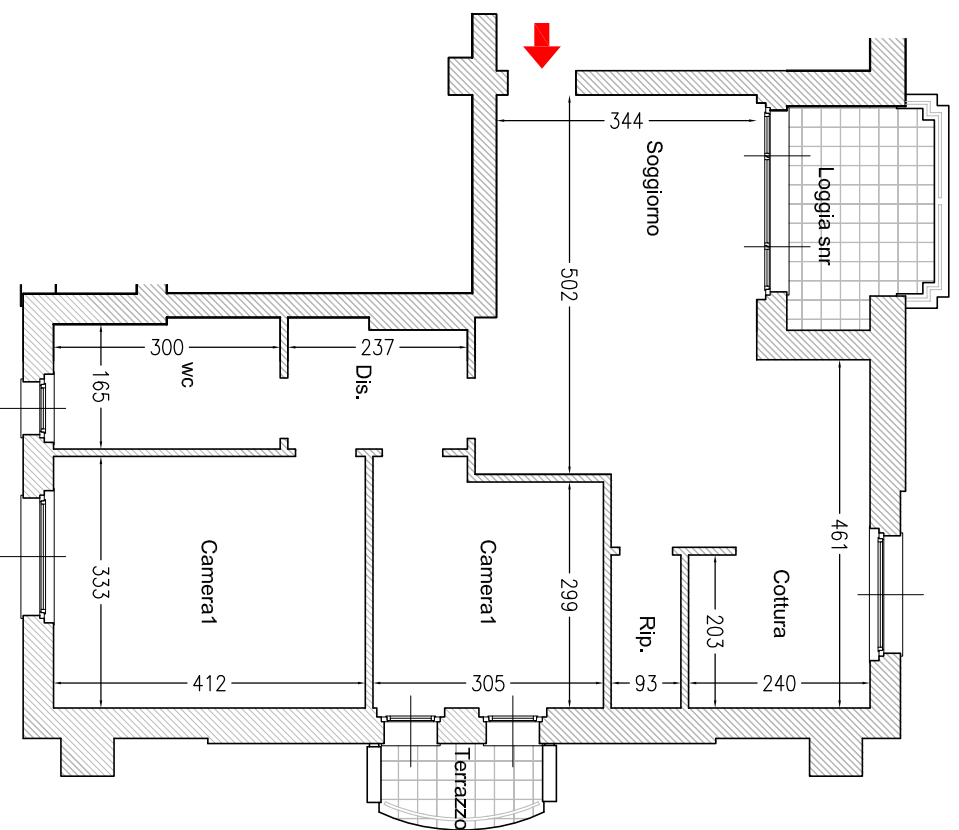
PIANO PRIMO
